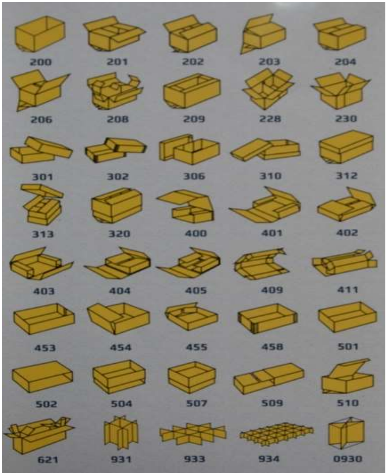
Cateva dintre modelele pe care utilajul le poate produce
